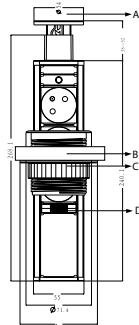
Рис.2 Технические размеры
