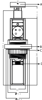
Rys.2 Wymiary Techniczne
