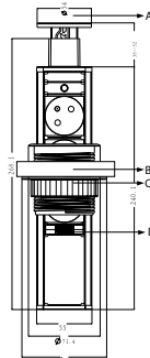
Obr.2 Technické rozměry
